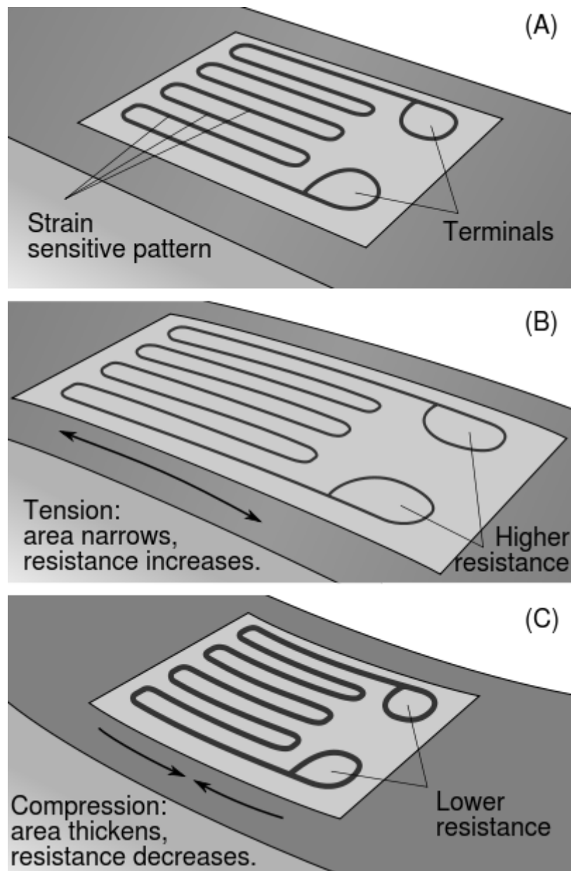
Рисунок 1 Пример датчика деформации
